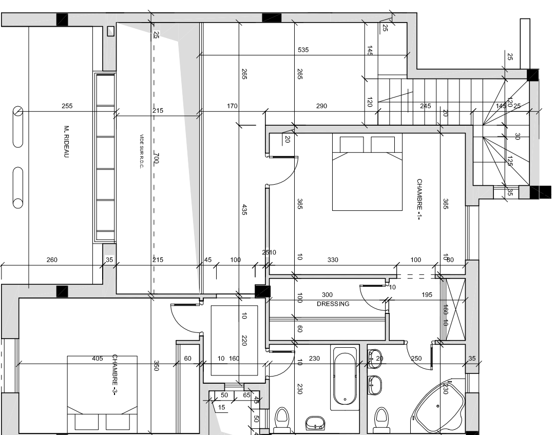
Plan ETAGE
