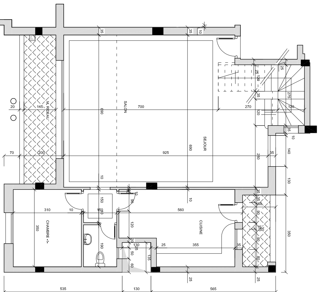
Plan RDC
